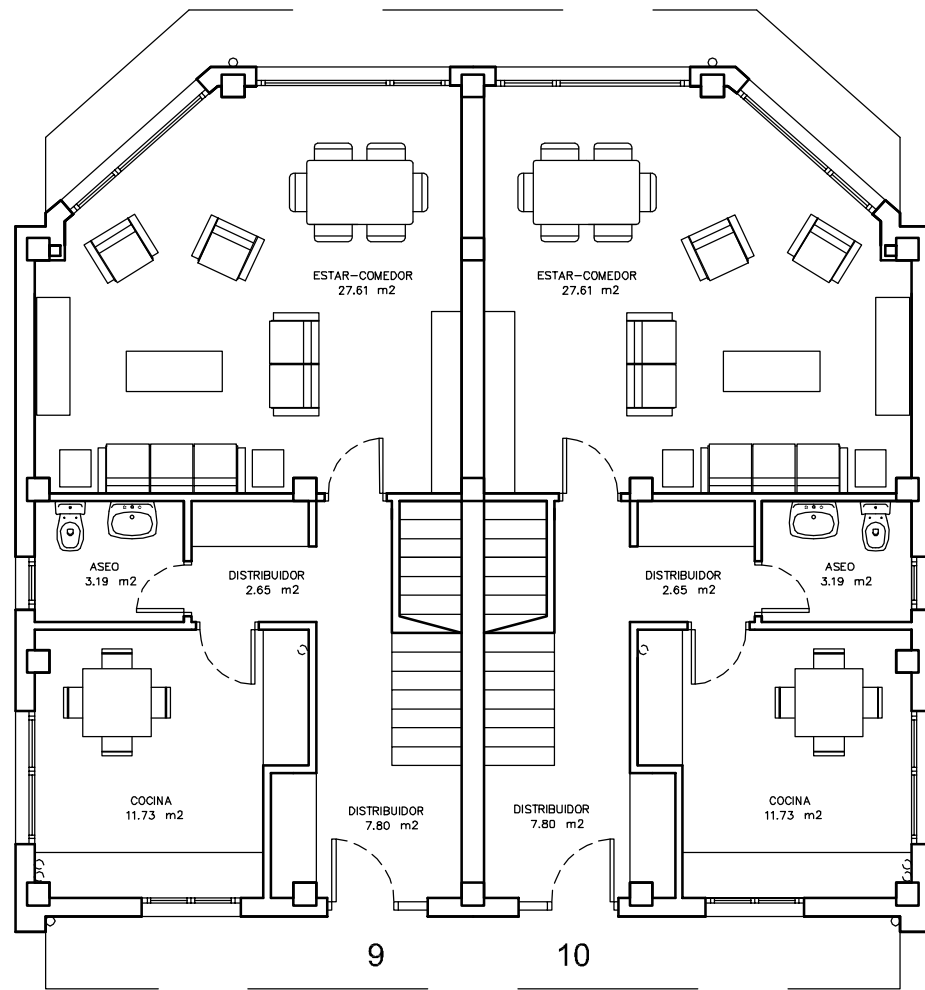
PLANTA BAJA Edificio 2
