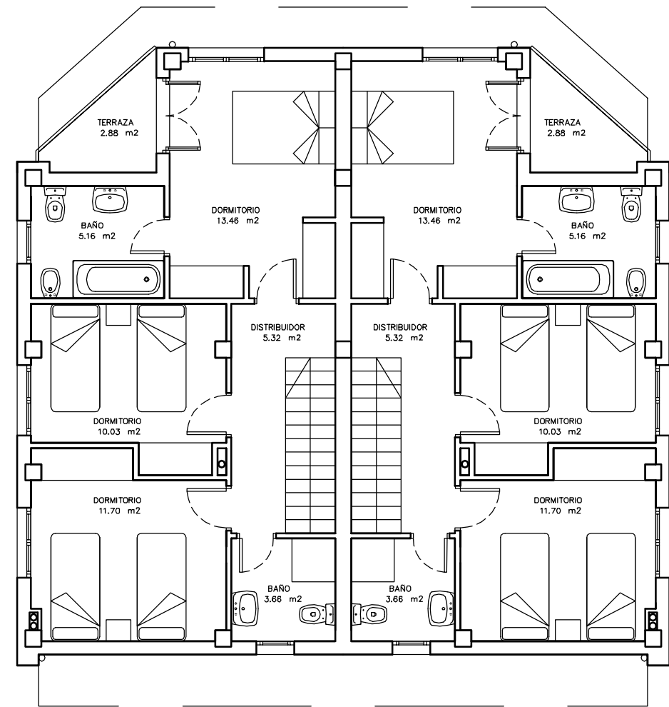
PLANTA PRIMERA Edificio 2
